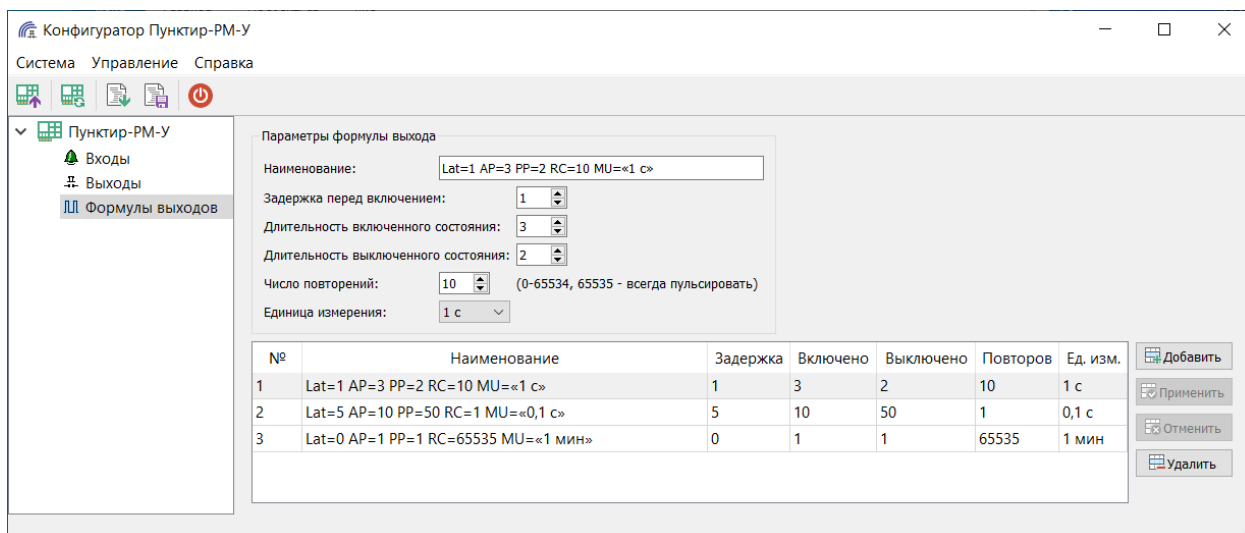
Рисунок 6 – Формулы выходов
